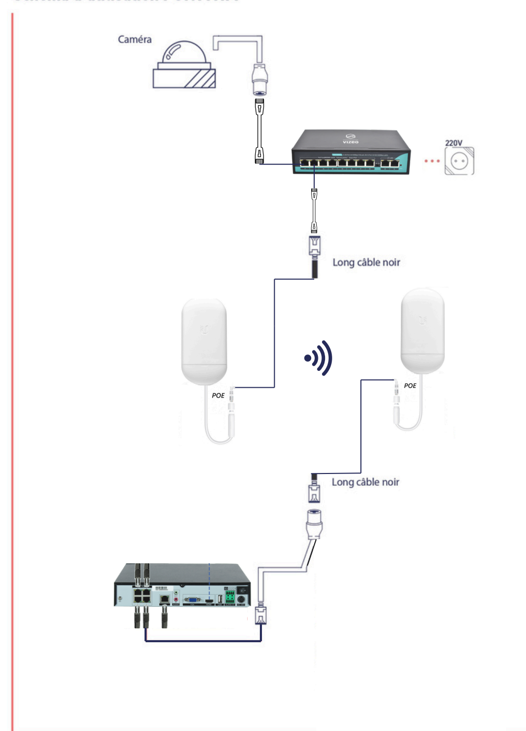
Schéma d'utilisation PONTWIFI
